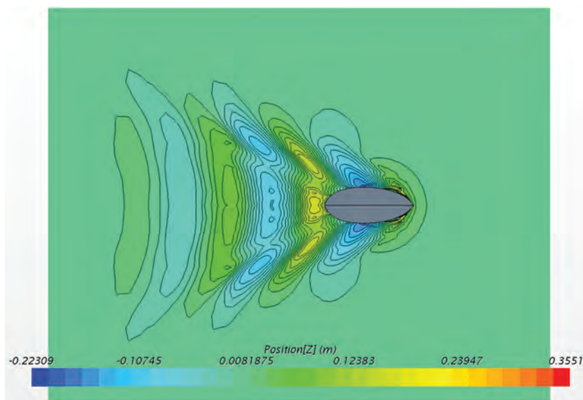
Figure 15 Wave pattern around the fishing vessel at V = 6 kn Slika 15. Slika valova oko ribarskog broda pri V = 6 čv
